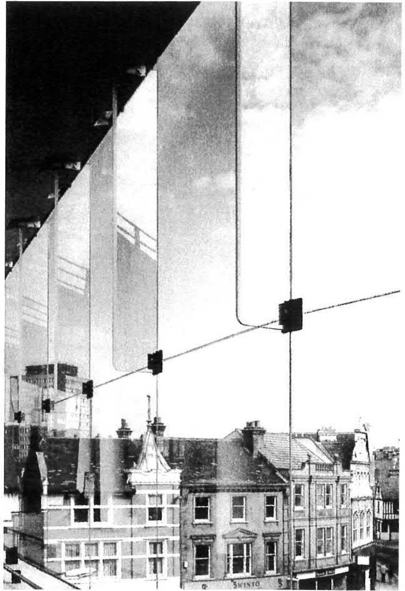
Peter Rice, Martin Francis und Ian Ritchie [RFR], Musée de la science im Parc de la Villette, Paris. Reyner Banham. «Luxe, calme et technicité». In: Architectural Review 1/1996, Vol. CLXXX, Nr. 1078
